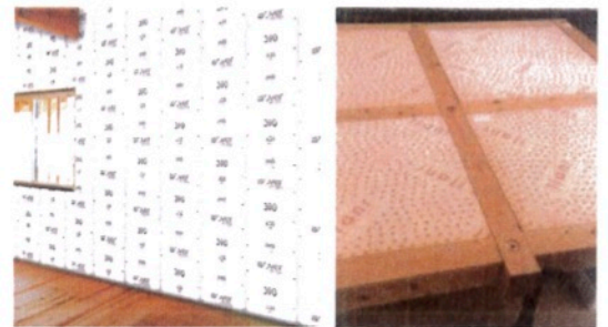
天井・壁/高性能グラスウール16k 床/フェノールフォーム
