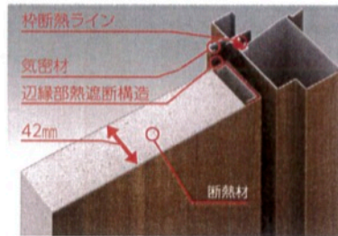
気密材断熱材辺縁部熱遮断構造枠断熱ライン42mm
